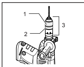
1. Base de mandril 2. Anillo 3. Mandril de cambio rápido
