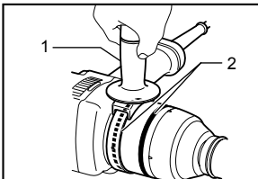
1. Side grip 2. Groove
